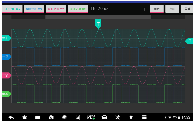
图 15-1 示波器界面
